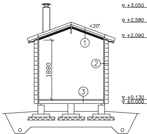
LEIKKAUS / SKÄRNING A - A
